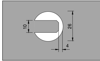
01.021.001.00 kantbescherm- profiel
