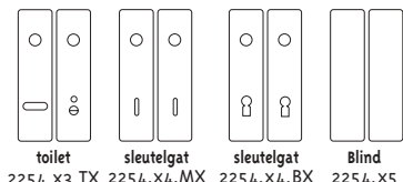
blind 2254.X0 cilinder 2254.X2.RX cilinder 2254.X2.EX cilinder 2254.X2.KX cilinder 2254.X2.UX
