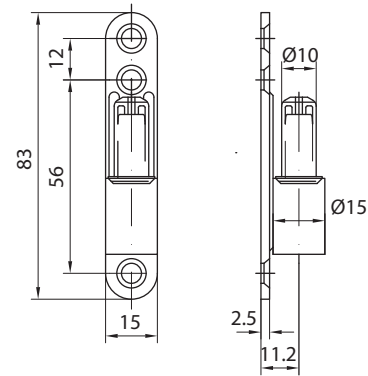
Fiche en applique réversible pour toutes huisseries bois, métalliques et aluminium, s'utilise avec les paumelles 4206 - V505.2 et caches fiches 4205 - V207 Reversible surface fixed butt for all types of wooden, metal and aluminium frame, to fit hinges 4206 - V505.2 and butt covers 4205 - V207
