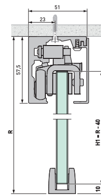
Portavant 60 Montage au plafond
