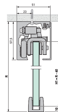
Portavant 60 Plafondmontage
