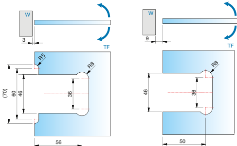
Usinages des verres pour les différents jeux d'écartement
